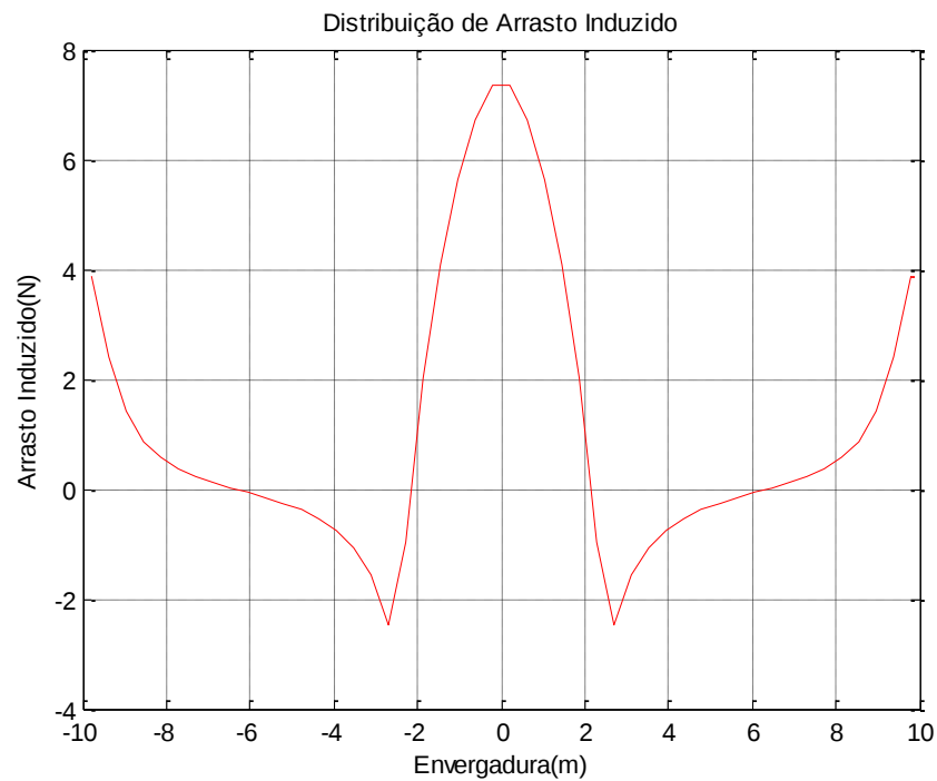
Figura 60: Distribuição de arrasto induzido para um enflechamento de 30°
