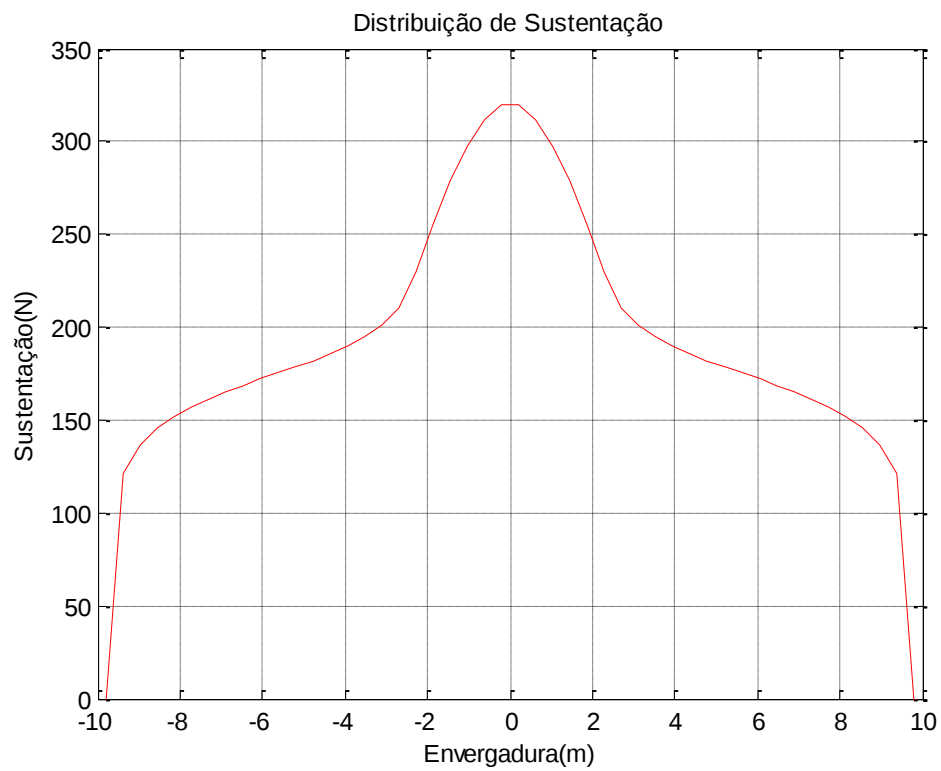
Figura 53: Distribuição de Sustentação para um enflechamento de 15°
