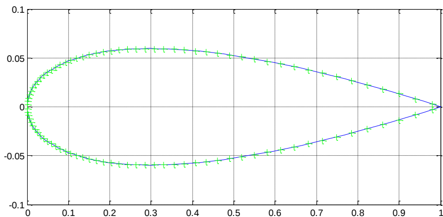
Figura 25: Discretização do fólho com os pontos de controle
