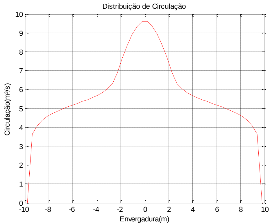
Figura 52: Distribuição de Circulação para um enflechamento de 15°
