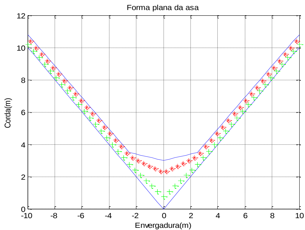
Figura 61: Asa traapezoidal com 45° de enflechamento com kink
