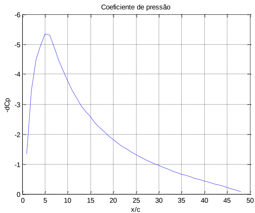
Figura 30: Distribuição da variação do coeficiente de pressão
